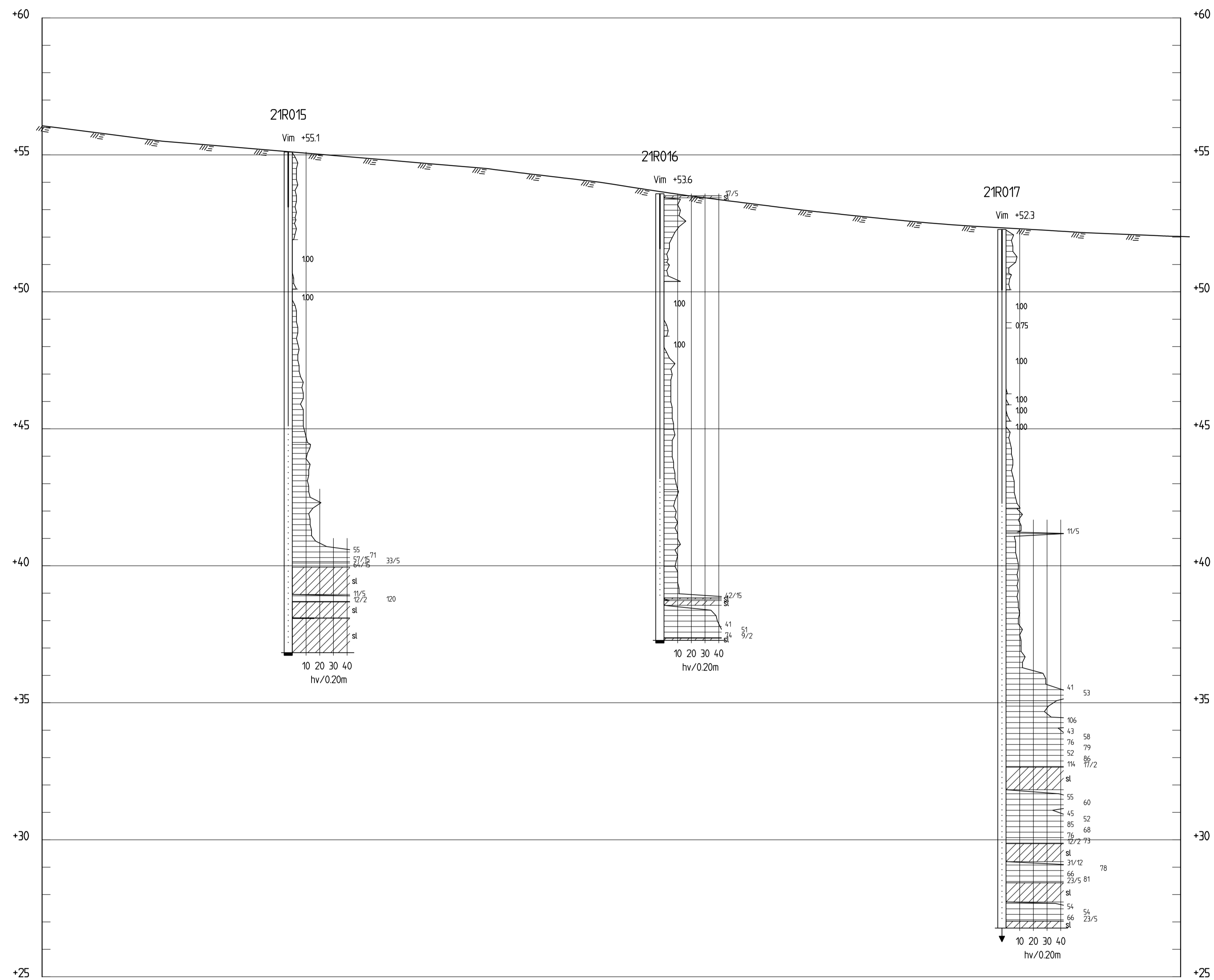
SEKTION P-P H 1: 100 L 1: 400
